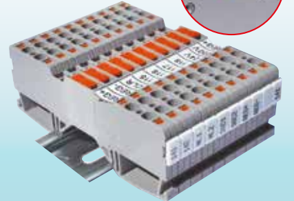
2 Giriş / 2 Çıkış Test Klemensi
