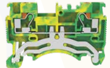
DS1.5-PE
