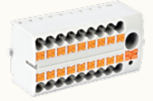
PMIT15 6-18x2,5
